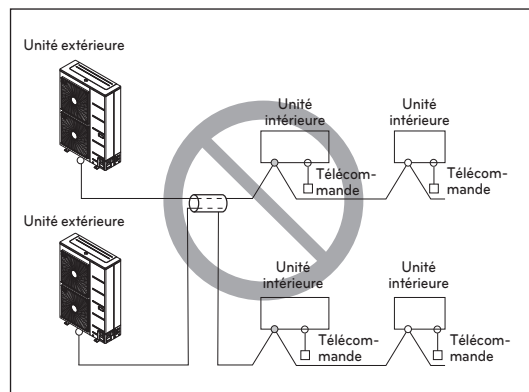
Câble multipolaire
