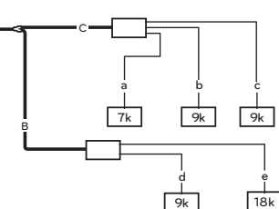
Ex) Modèles à distributeur 1Ø, 40kBtu/h
