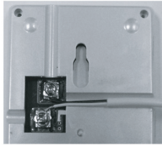
Fixation de la sonde à distance
