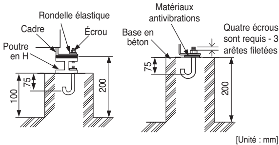
Méthode de fixation du boulon d'ancrage
