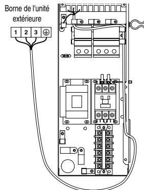
Résistance chauffante 30
