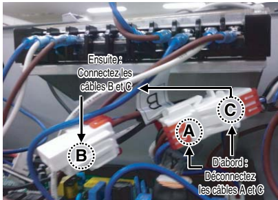
Résistance chauffante 30
