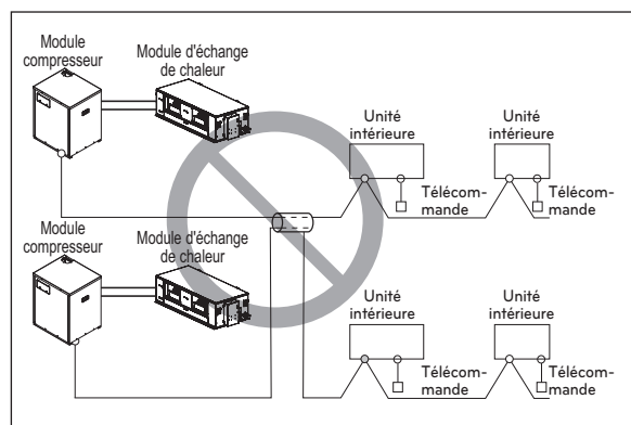
Câble multipolaire
