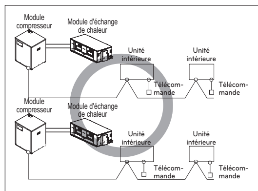
Câble bipolaire blindé
