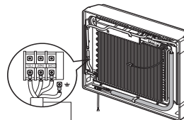
Câble d'interconnexion
