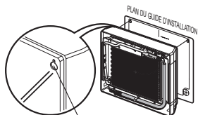
Trou de suspension (face arrière du produit)
