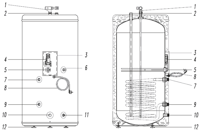
Ballon d'eau sanitaire (chauffage thermique solaire pris en charge)
