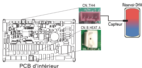
(Pour l'unité intérieure Split R32 Série 4, Pour l'unité intérieure Split R410A Série 3)
