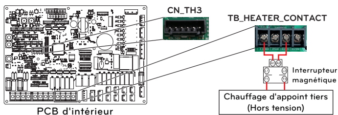
PCB d'intérieur
