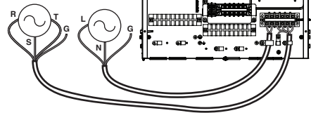
Chauffage d'appoint 3Ø (pour Hydrosplit)
