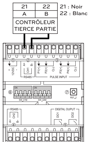
Interface du compteur
