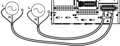
Chauffage d'appoint 1Ø (pour Hydrosplit)
