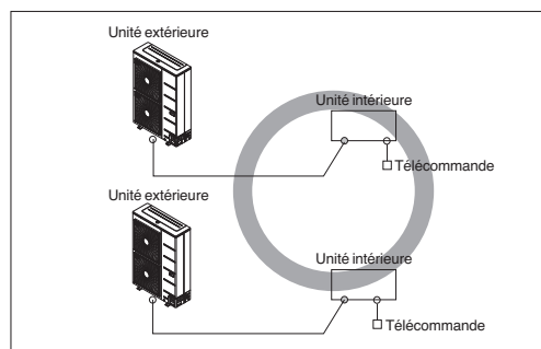
Câble blindé à deux conducteurs
